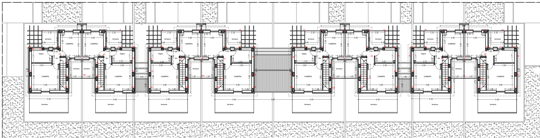
PIANTA PIANO PRIMO scala 1:100
